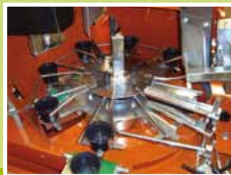
Réglage simultané des 8 supports de pots.
